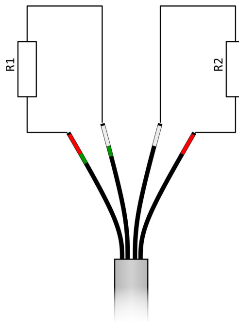
Obrázek 10.7: 2 x RTD v dvouvodičovém zapojení
